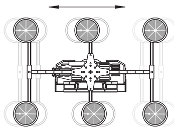
300mm (12") side shift
